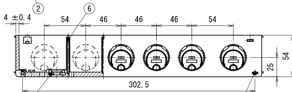
A-A 断面図
